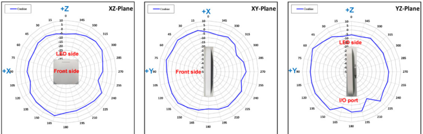
5 GHz Antenna
